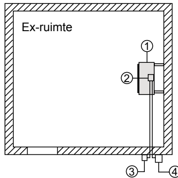
Bovenaanzicht
