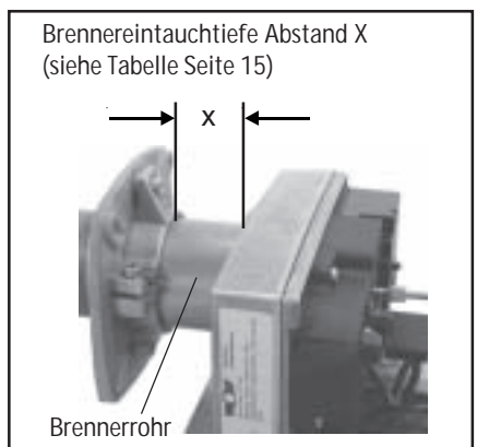
Bild: Brennereintauchtiefe
