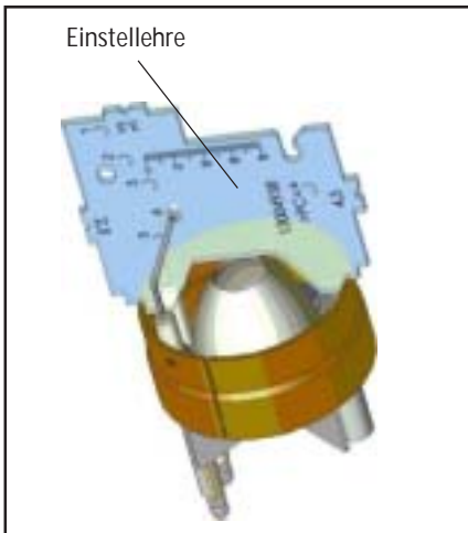
Bild: Einstellehre
