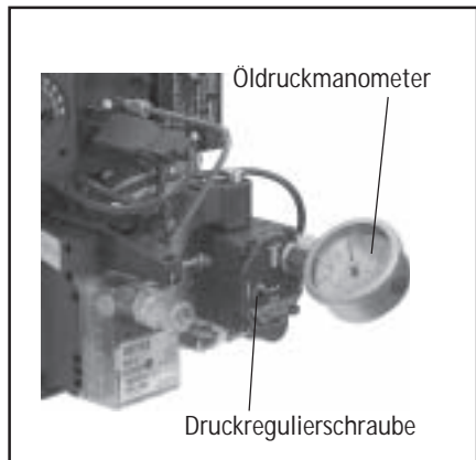
Bild: Öldruckmanometer
