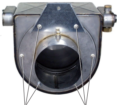
Flanschbefestigungsschrauben demontieren
