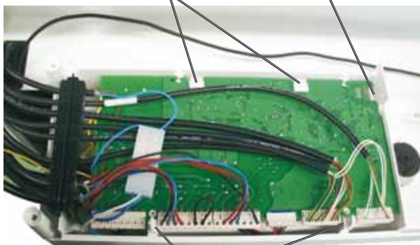
Zatrzaski do mocowania płytki
