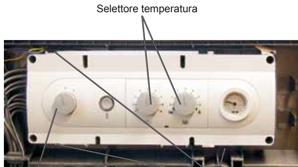
Interruttore di esercizio ON/OFF Regolazione linguette d'aggancio
