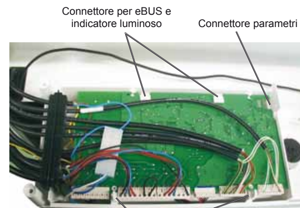
Linguette d'aggancio per fissare la scheda
