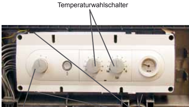
Betriebsschalter EIN/AUS
