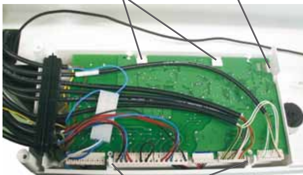
Защелки для фиксации платы
