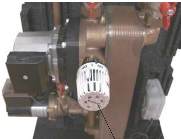
Régulateur thermique à valeur fixe
