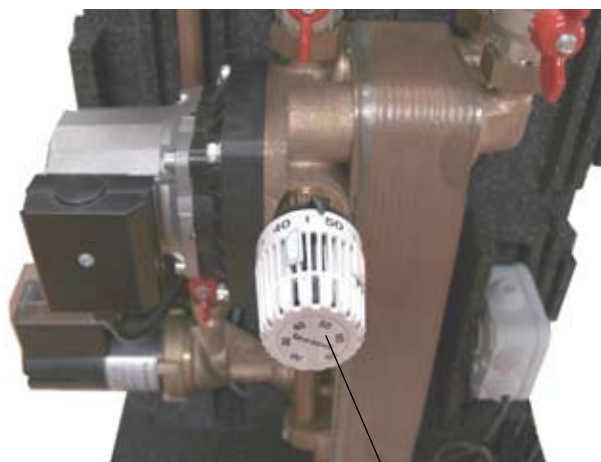
tepelný regulátor s konstantně nastavenou teplotou
