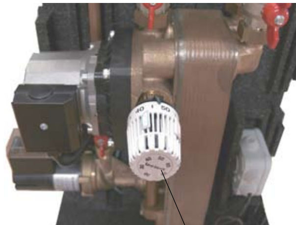
Θερμοστατική κεφαλή σταθερής ρύθμισης
