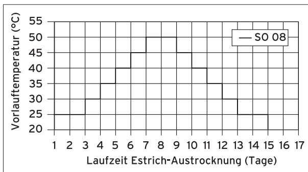
Abb. 6.1 Zeitlicher Verlauf automatisches Estrich austrocknungsprogramm (Parameter SO08 = 50 °C)
