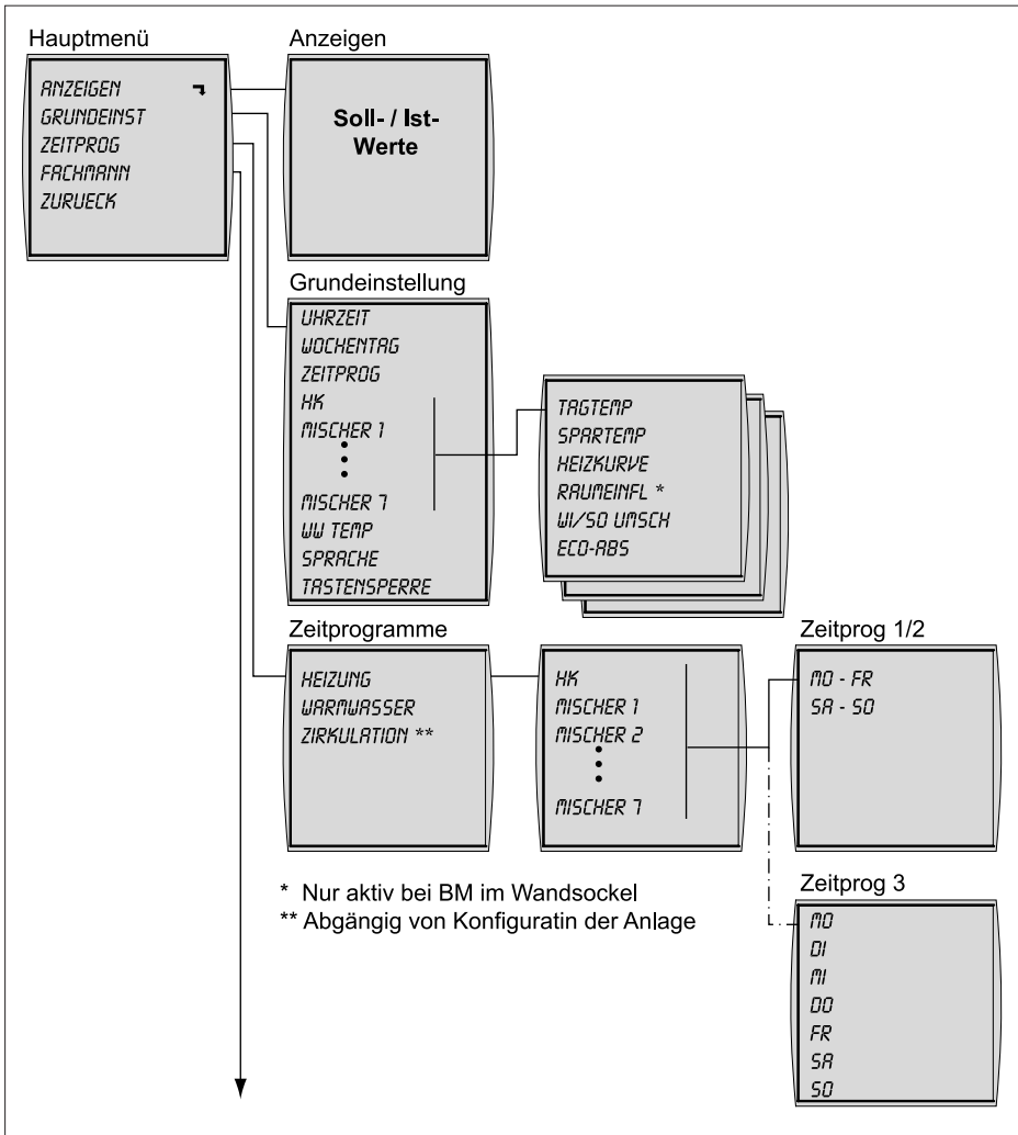
Abb. 5.2 Menüstruktur Bedienmodul BM
