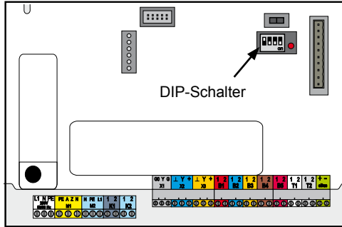
Regelungsplatine
