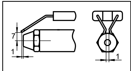
Bild: Elektrodenabstand
