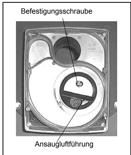
Bild: Ansaugluftführung
