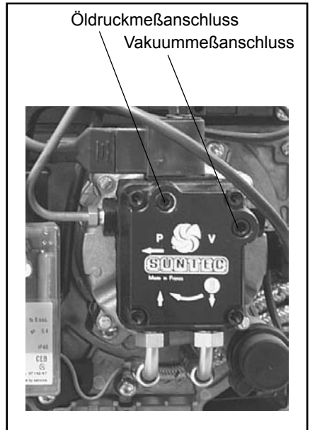
Bild: Unterdruckkontrolle
