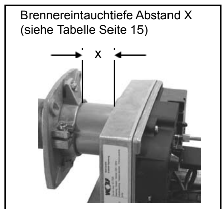
Bild: Brennereintauchtiefe
