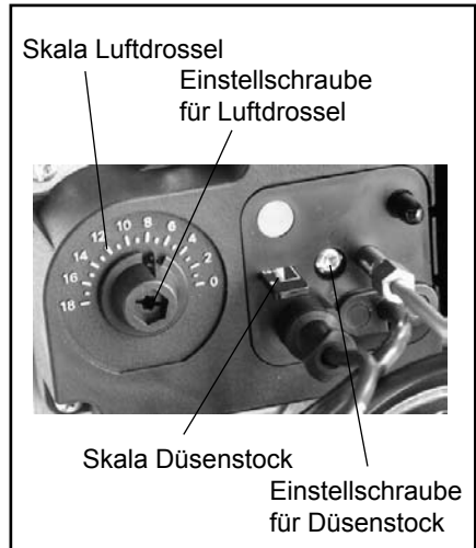
Bild: Luftregulierung
