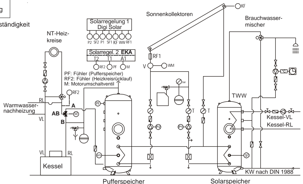
Anlagenschema 2.0 Solare Warmwasserbereitung und Raumheizungs-Unterstützung
