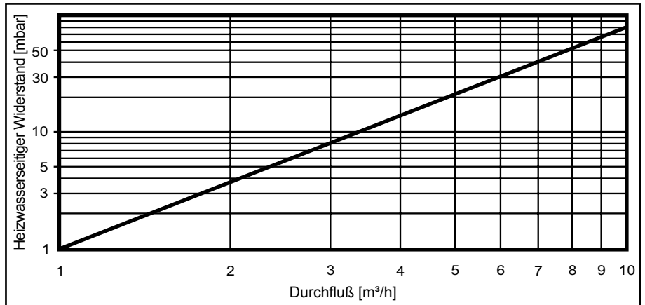
Bild: Heizwasserwiderstand
