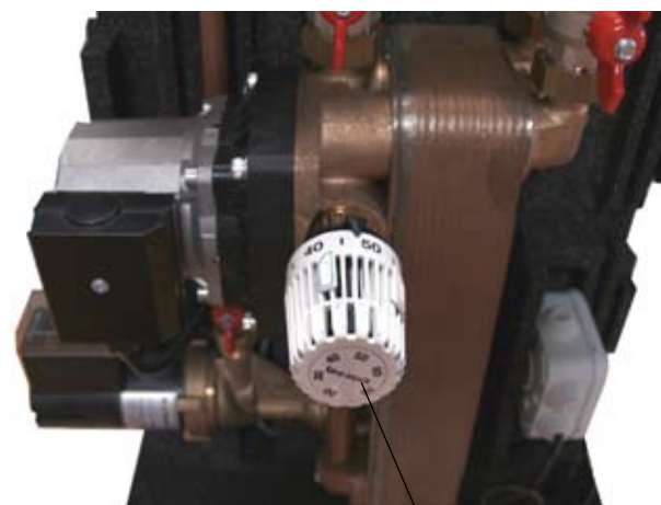
Maximaalthermostaat
